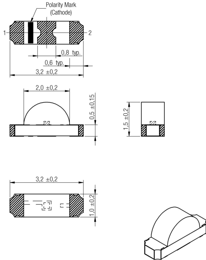
Scale - 10:1
